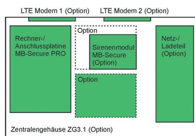
Zentralengehäuse ZG3.1
