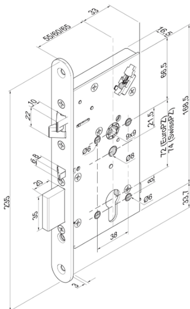
Maßzeichnung Vollblatt
